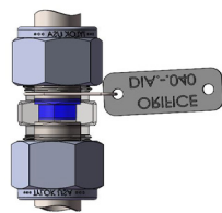
ORIFICE INSERT pp. 72
